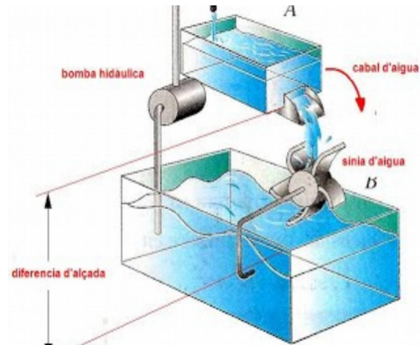
Circuit d'aigua
